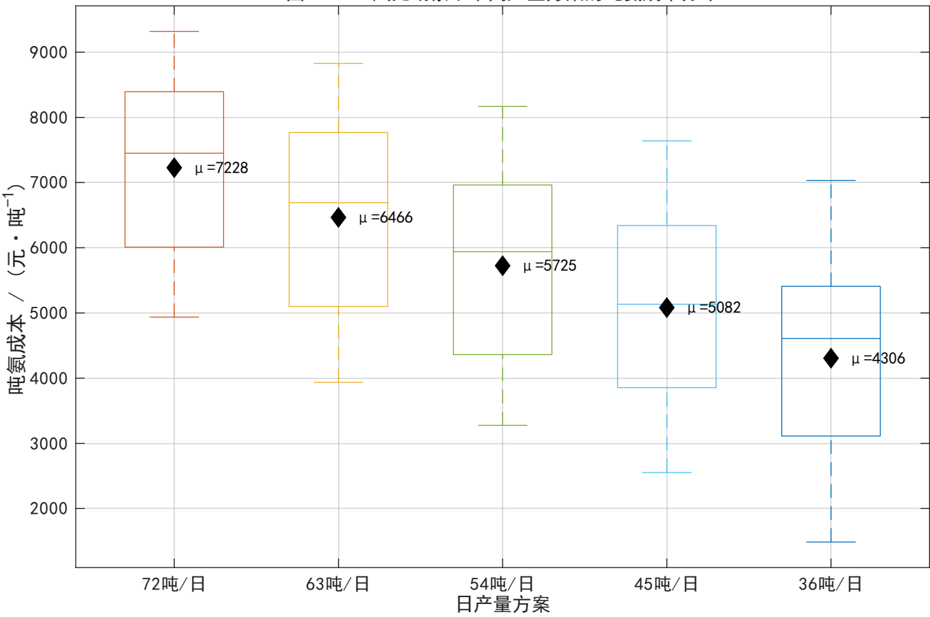
图 2 24 风光场景下不同产量方案的吨氨成本分布
